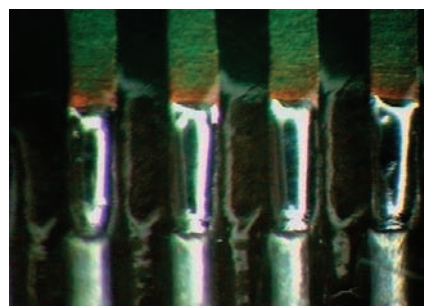
잔사 및 솔더링 특성 우수 (Excellent Soldering and Residue Properties)
