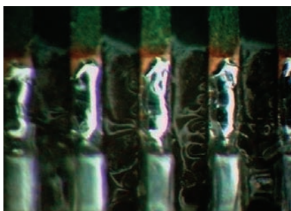
잔사 버블 발생 (Residue Bubble)
